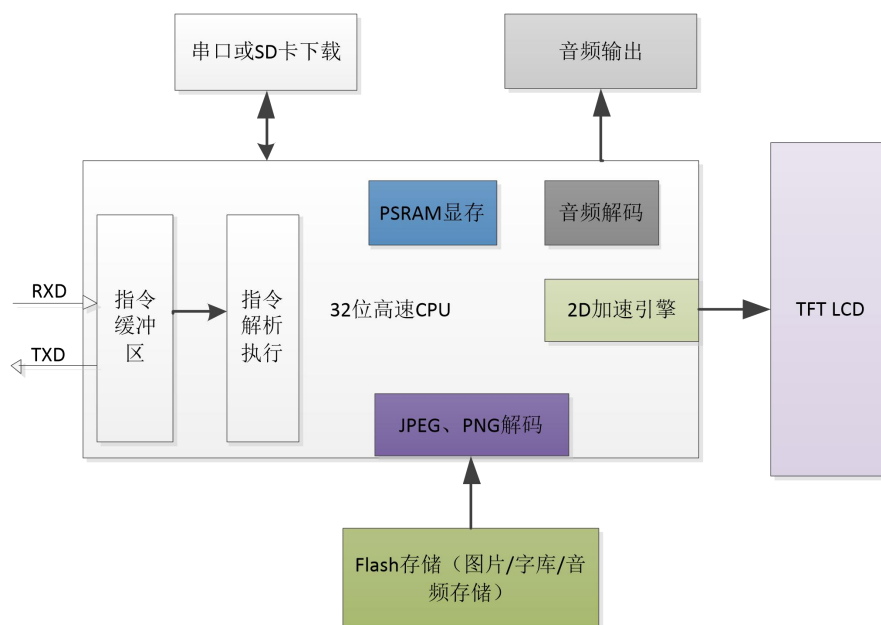
图 2-1 DN 系列串口屏内部结构图
