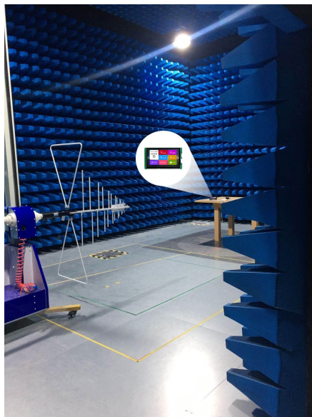
图 5-5 辐射测试图
