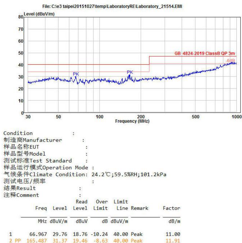
图 5-7 辐射测试垂直方向
