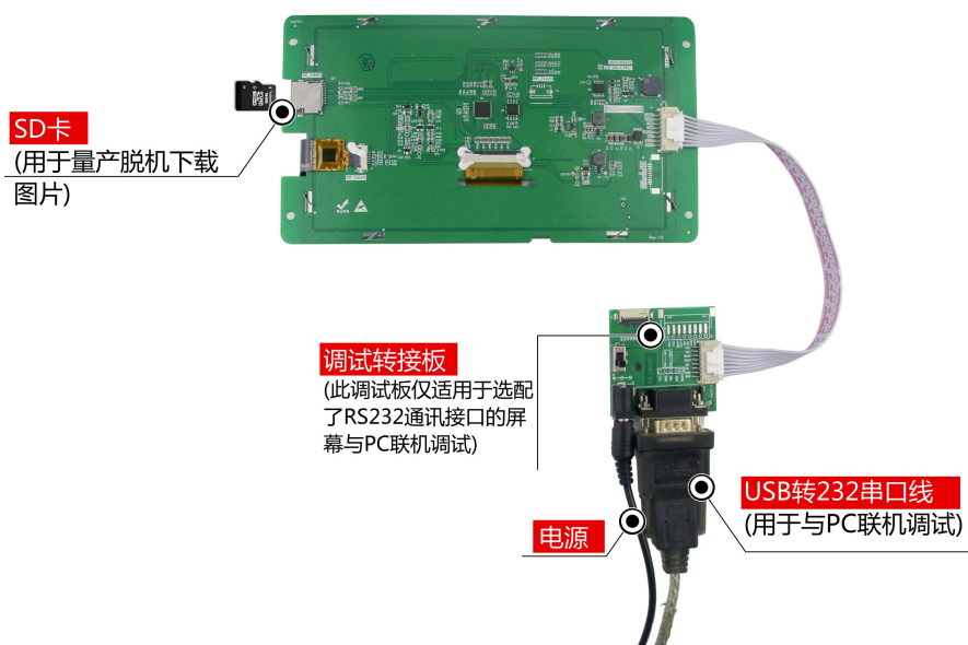
图 1-5 调试工具图
