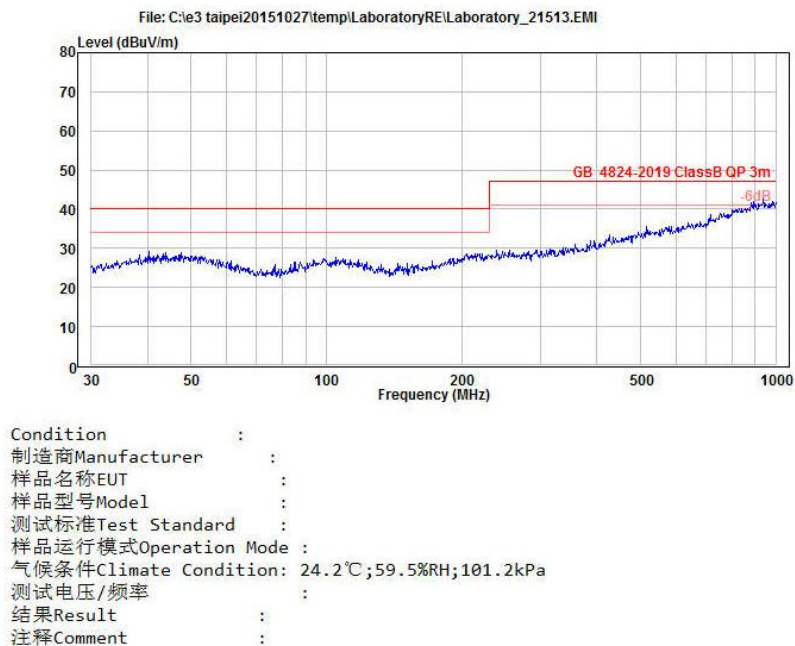
图 5-6 辐射测试水平方向
